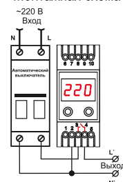
Монтажная схема
