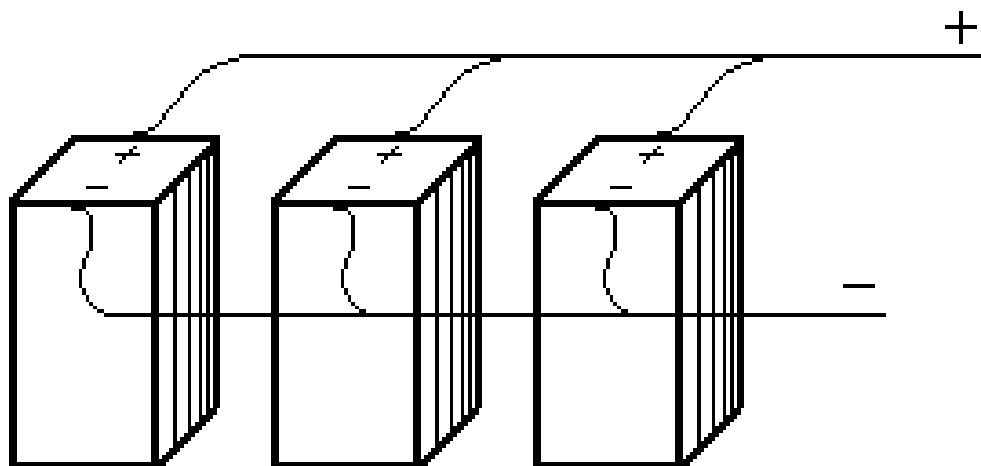
Рис.2. Пример параллельного соединения нескольких 12В батарей для получения 12В
