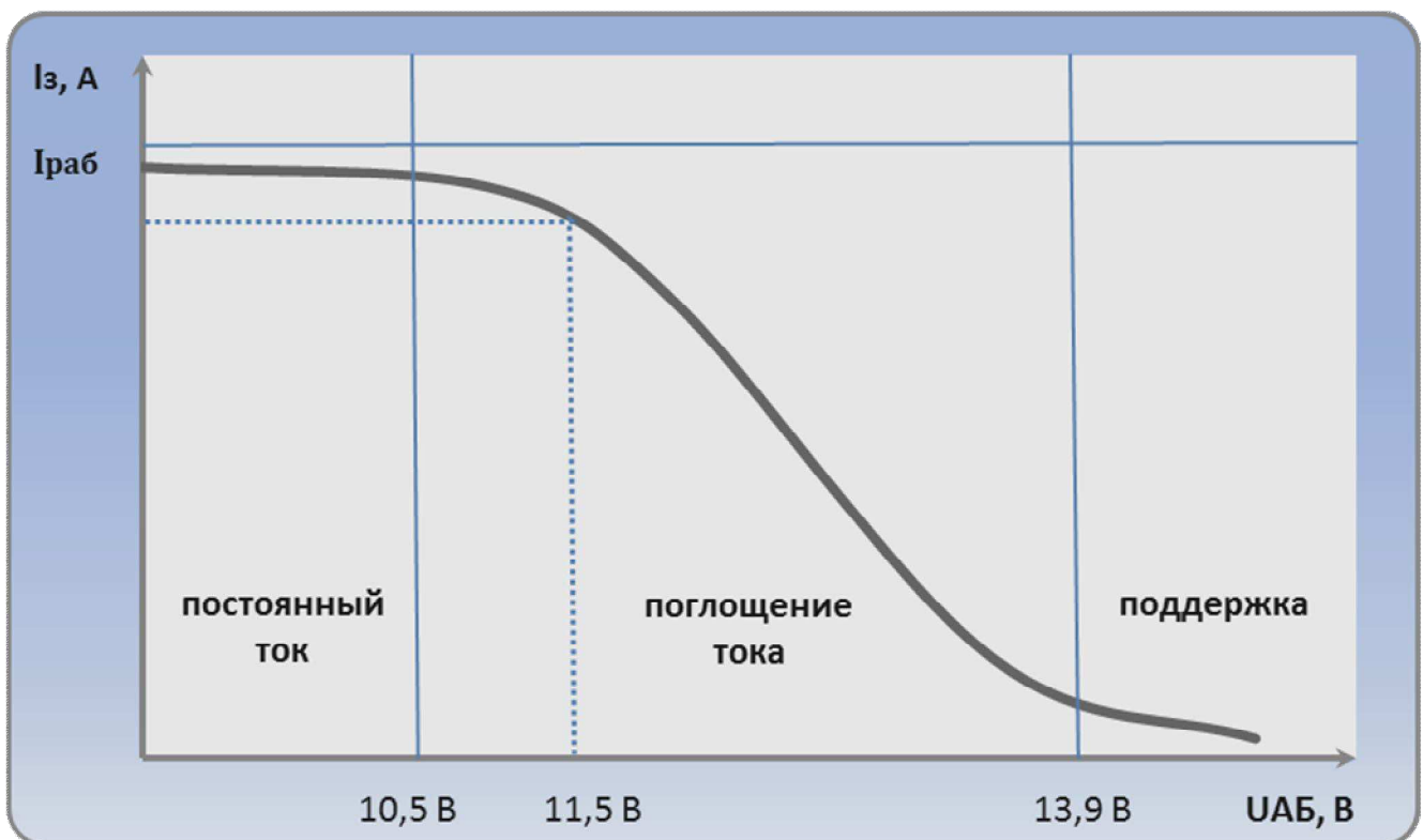
Рис.4. График работы зарядного устройства. Улучшенный заряд по Вубриджу (трехстадийный режим заряда)
