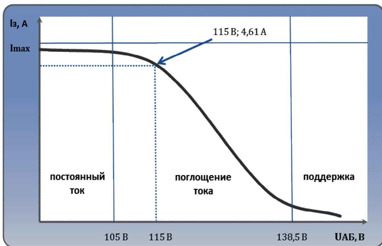
Рис.9. График работы зарядного устройства. Улучшенный заряд по Вубриджу (трехстадийный режим заряда)
