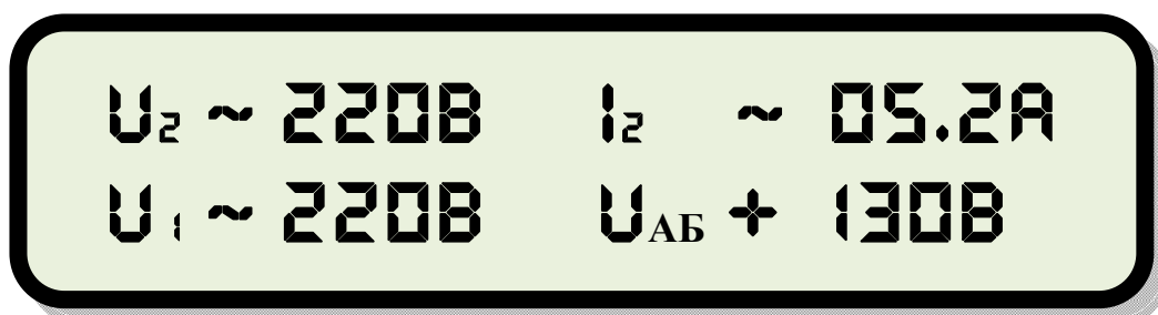
Рис.7. Индикатор на передней панели ИБП, где: U_1 – 220В (напряжение входящей сети); U_2 – 220В (напряжение на выходе ИБП); U_{AB} – 130В (напряжение на АКБ при работе зарядного устройства); I_2 – 05.2А (ток потребляемый проверочной нагрузкой);
