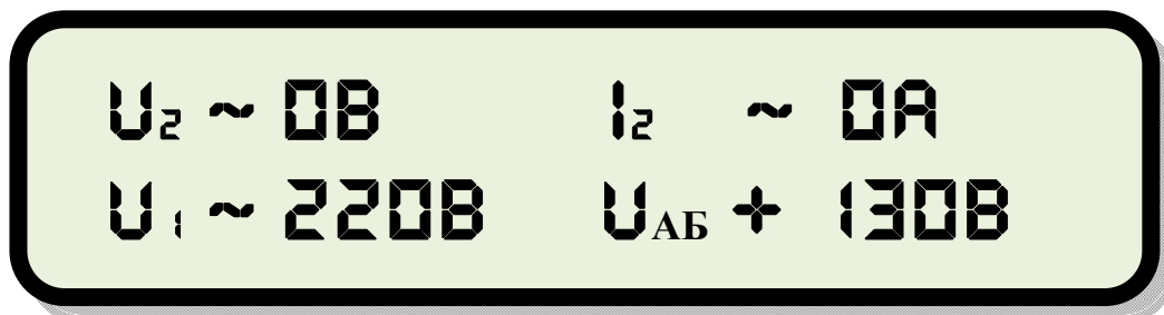
Рис.6. Индикатор на передней панели ИБП, где: U_1 – 220В (напряжение входящей сети); U_2 – 0В (на выходе ИБП нет напряжение); U_{AB} – 130В (напряжение на АКБ при работе зарядного устройства); I_2 – 0А (нагрузка не подключена);
